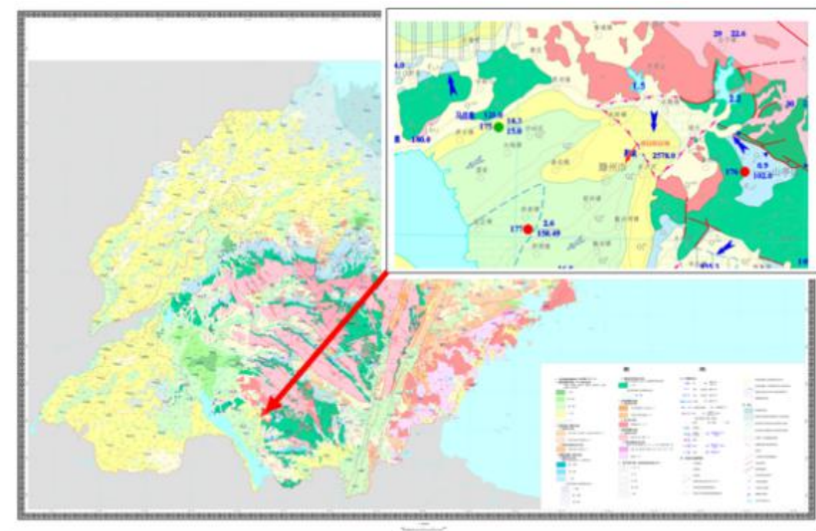
图 3.1-1 水文地质图
